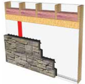
Charpente standard avec OSB ou contreplaqué et isolant rigide
